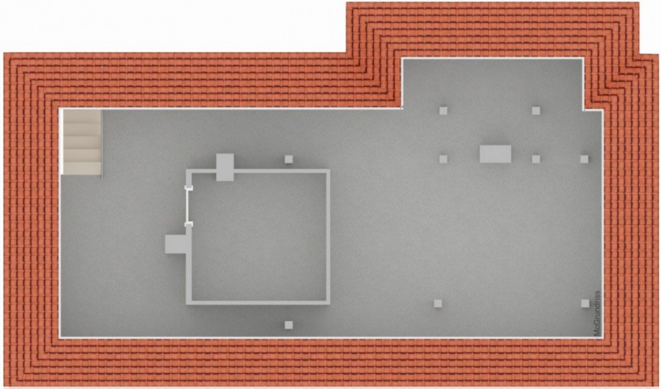
Grundriss - DG
